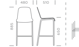
Tubo Tube Ø16
